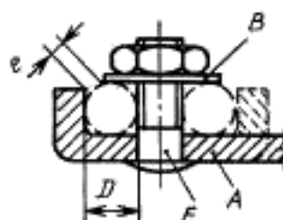
Болтовые зажимы
