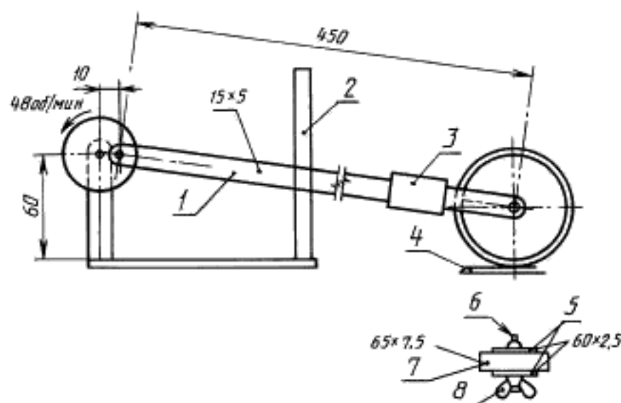
Рисунок 6* — Устройство для вдавливания шарика
