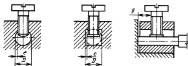
Рисунок 11 — Колонковые зажимы, лист 1
