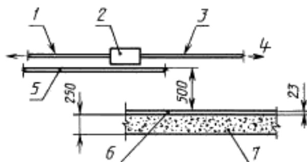
Рисунок 4 — Испытание на удар отдельно стоящих управляющих устройств
