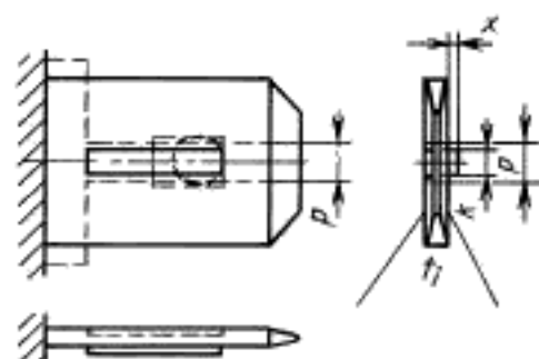
Рисунок 14 — Ответная часть зажима (лепесток), лист 3
