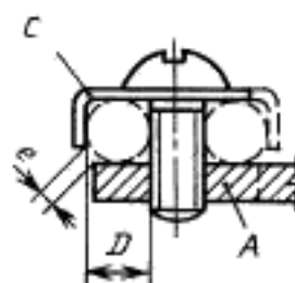
Винтовые зажимы
