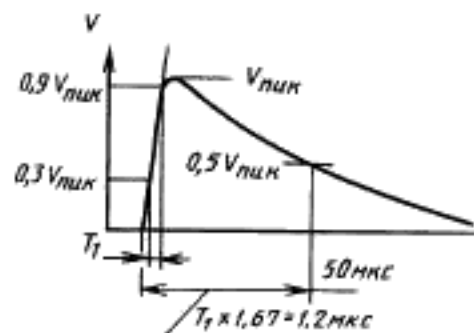
Рисунок Н.26.8.1 — Форма волны при разомкнутой цепи
