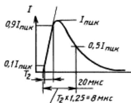
Рисунок Н.26.8.2 — Форма волны тока разряда
