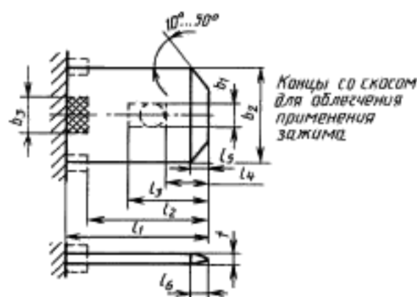
Рисунок 14 — Ответная часть зажима (лепесток), лист 1
