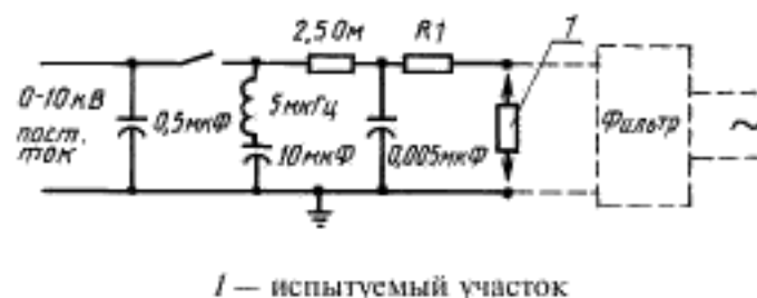
Рисунок Н.26.10.2 — Схема генератора ударных волн 0,5 мкс/100 кГц
