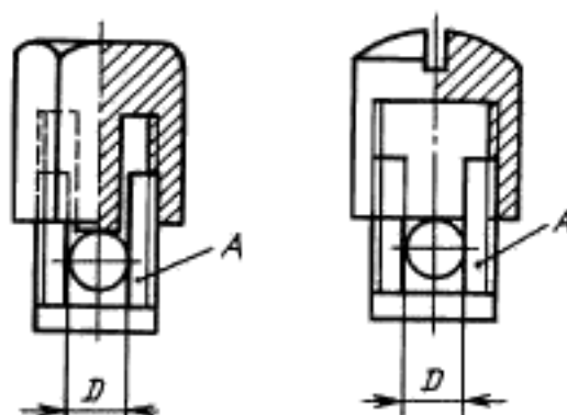
A — закрепленная часть; D — пространство для провода
