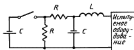
Рисунок Н.26.8.3 — Схема «гибридного» генератора
