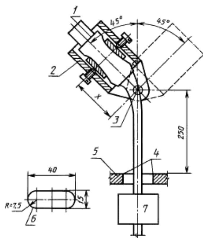
Рисунок 8 — Устройство для проверки стойкости маркировки к истиранию
