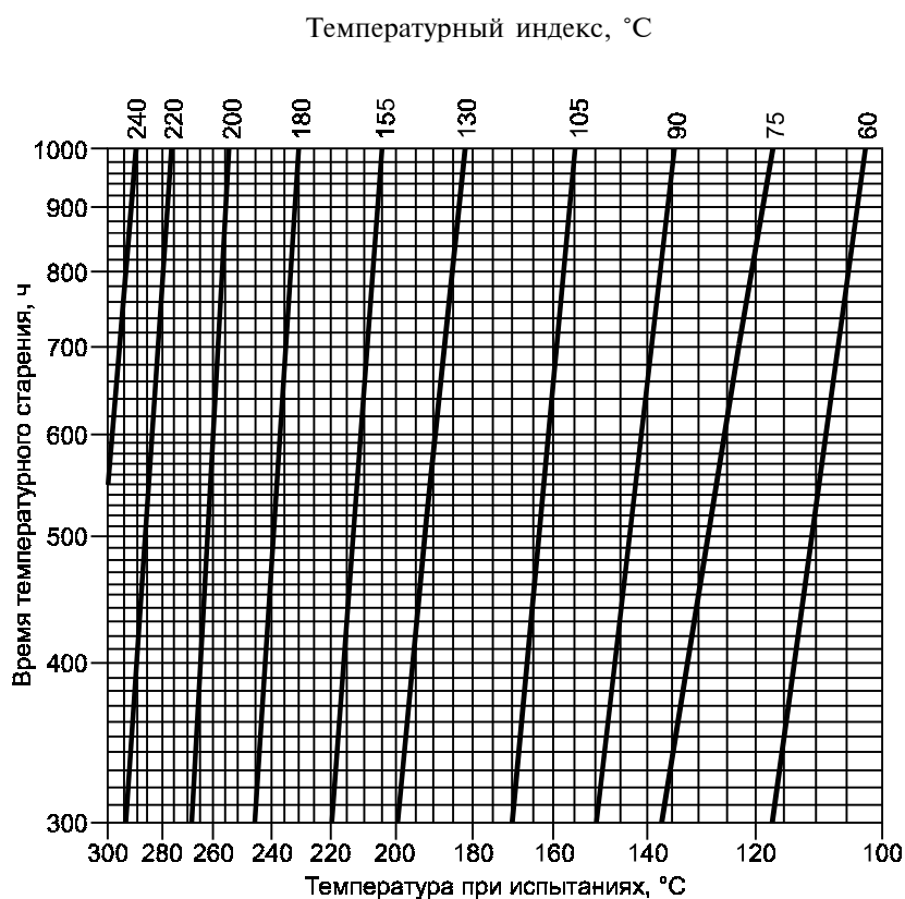
Рисунок 2G — Время теплового старения
