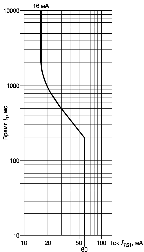
Рисунок М.2 — Кривая предельного значения тока I_{TS1} модулированного сигнала звонка
