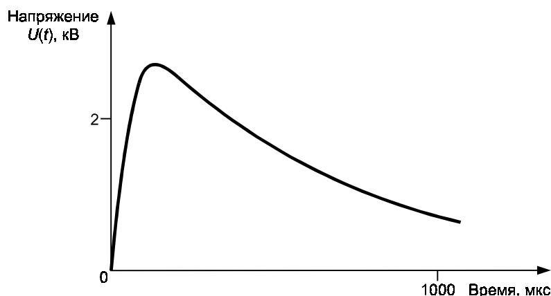
Рисунок S.1 — Форма сигнала при испытании изоляции (ограничитель выбросов отсутствует, пробоя изоляции нет)
