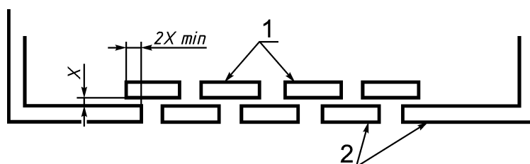
Рисунок 4F — Конструкция отражающей пластины
