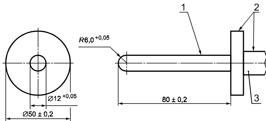
Рисунок 2С — Испытательный калибр
