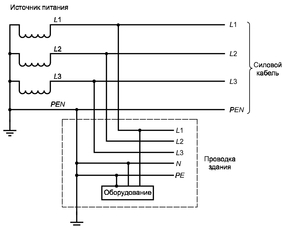
Рисунок V.2 — Пример TN-C-S системы энергоснабжения
