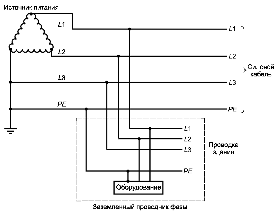
Рисунок V.1 — Пример TN-S системы энергоснабжения
