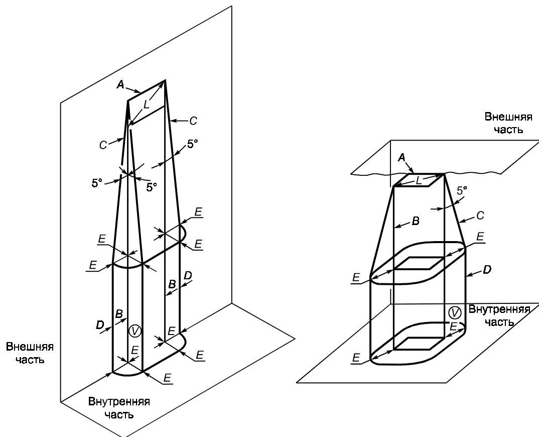
Рисунок 4С — Примеры конструкции жалюзи
