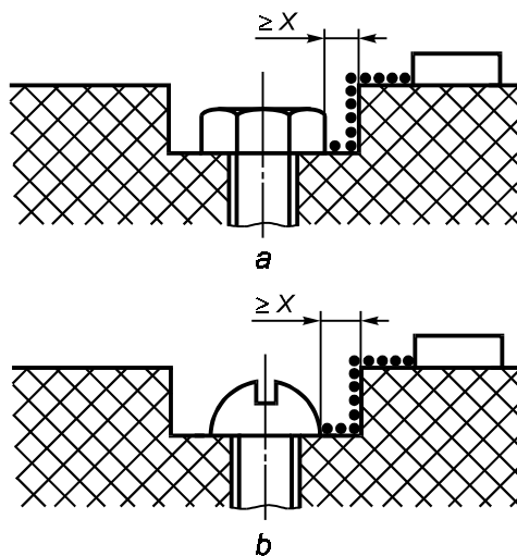
Рисунок F.9 — Широкое углубление
