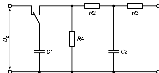
Рисунок N.1 — Схема генератора импульсов
