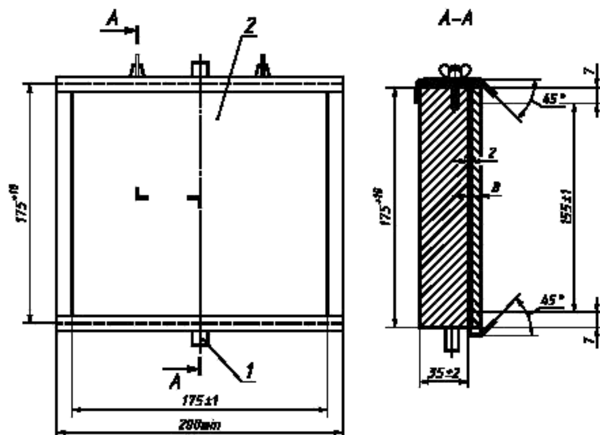
Рисунок 24 — Монтажная опора
