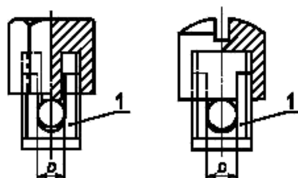
1 — неподвижная деталь; D — место расположения проводника 1
