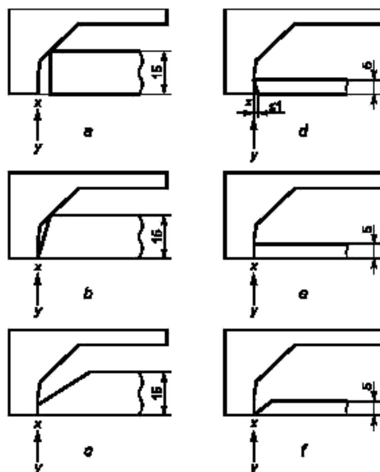
Рисунок 34 — Калибр для проверки габаритов крышек или закрывающих пластин (накладок)
