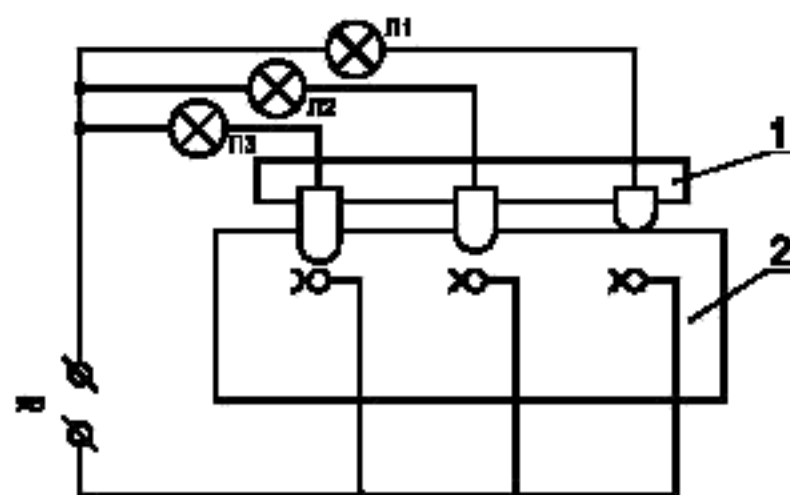
1 — вилка; 2 — розетка
