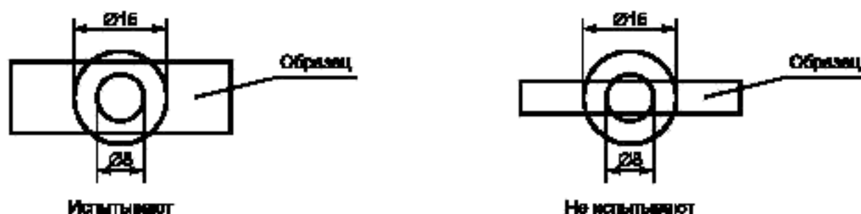
Рисунок 43 — Схематическое изображение требований 28.1.1
