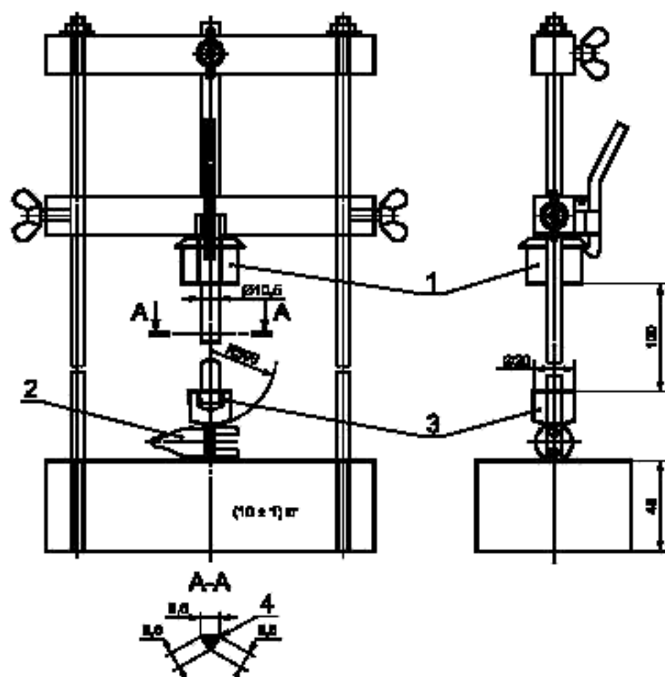
1 — боек массой (1000 \pm 2) г; 2 — образец; 3 — прижим массой 100 г; 4 — края закруглить
