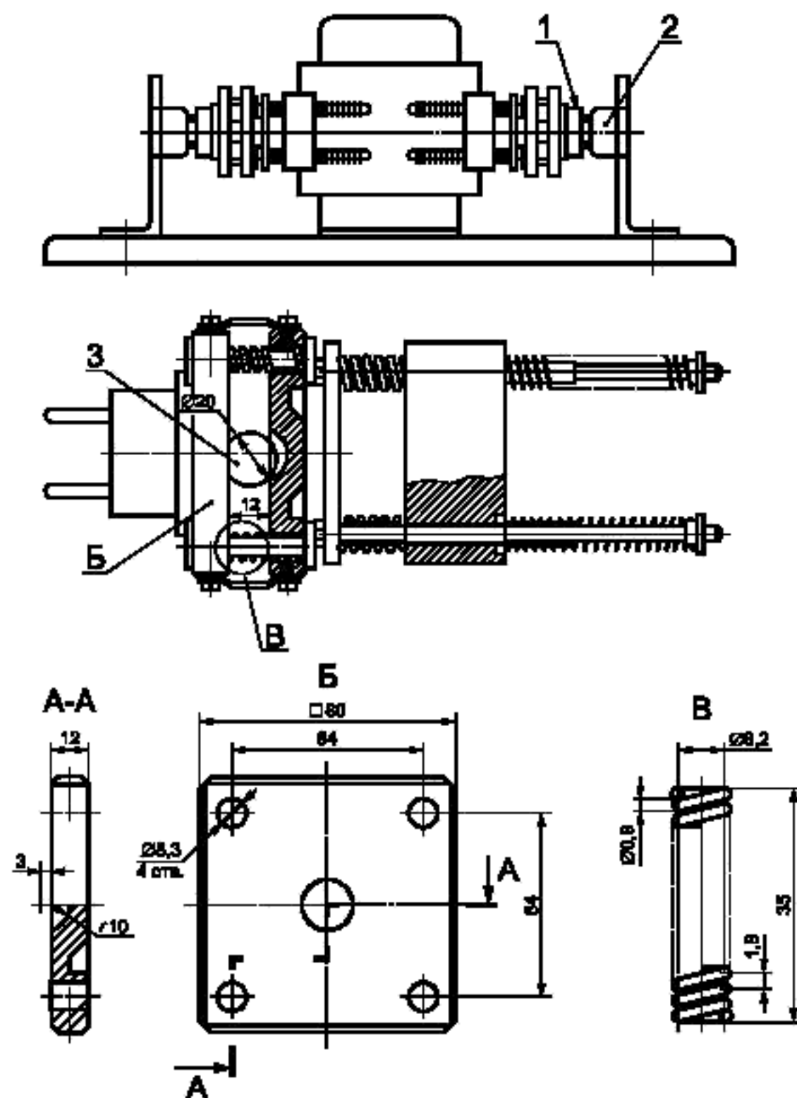
1 — вилки; 2 — розетка; 3 — стальной шар
