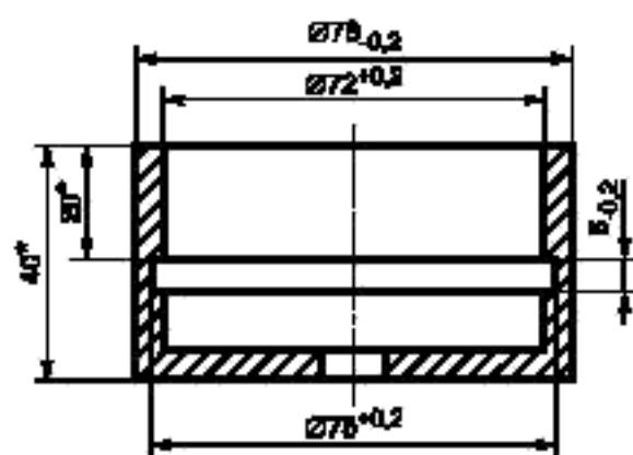
Рисунок Б.5 — Схема для проверки соединителей с заземляющим контактом на опережающее включение заземляющего контакта
