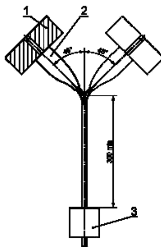
1 — устройство для закрепления образца; 2 — образец; 3 — груз
