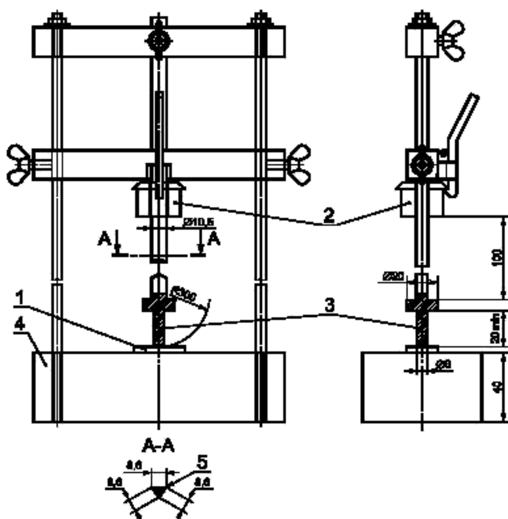
Рисунок 41 — Установка для испытания давлением при высокой температуре
