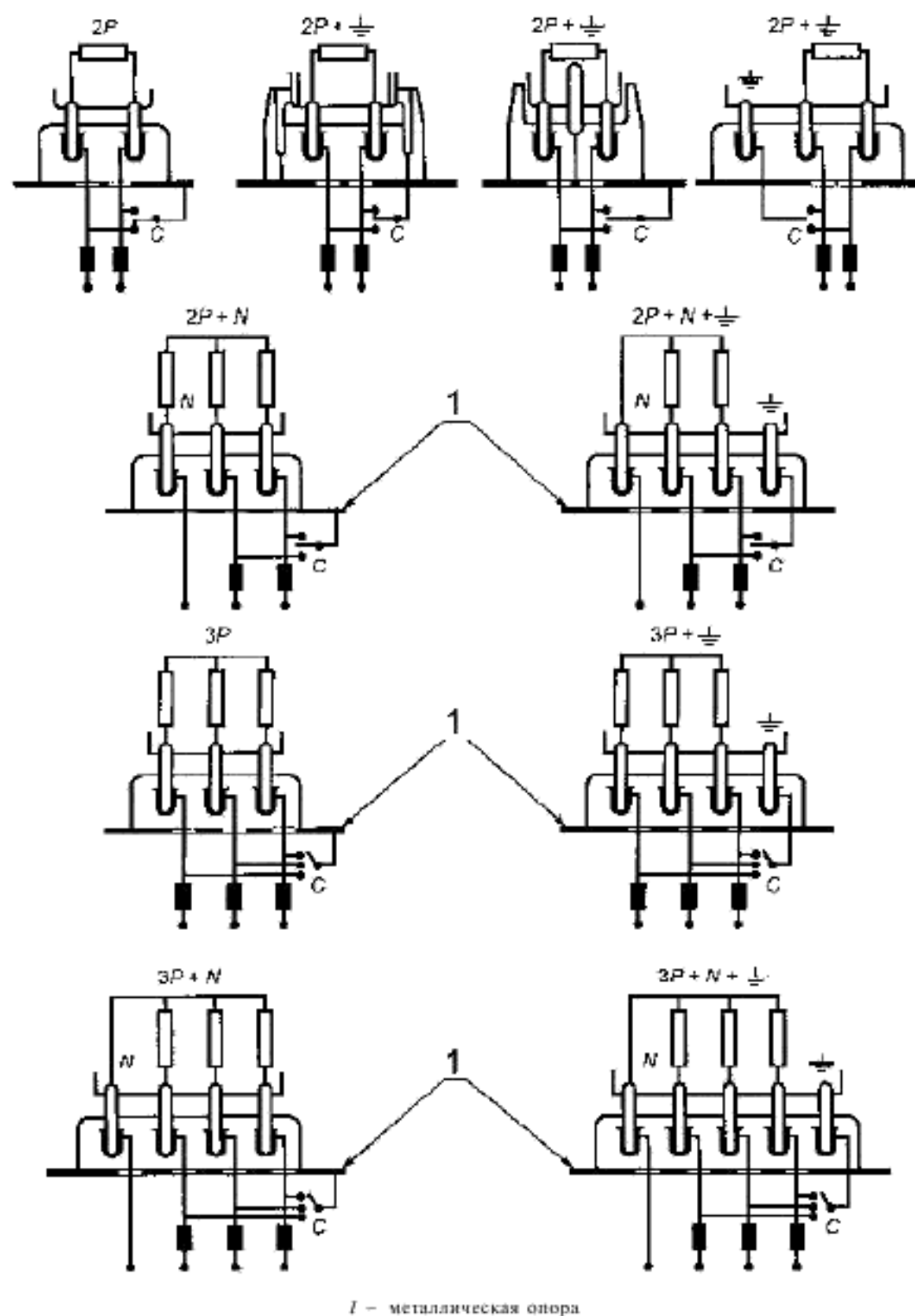
Рисунок 17 — Схемы соединения для испытания на нормальную работу
