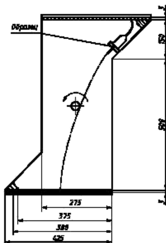
Рисунок 26 — Барабан для испытания соединителей на свободное падение
