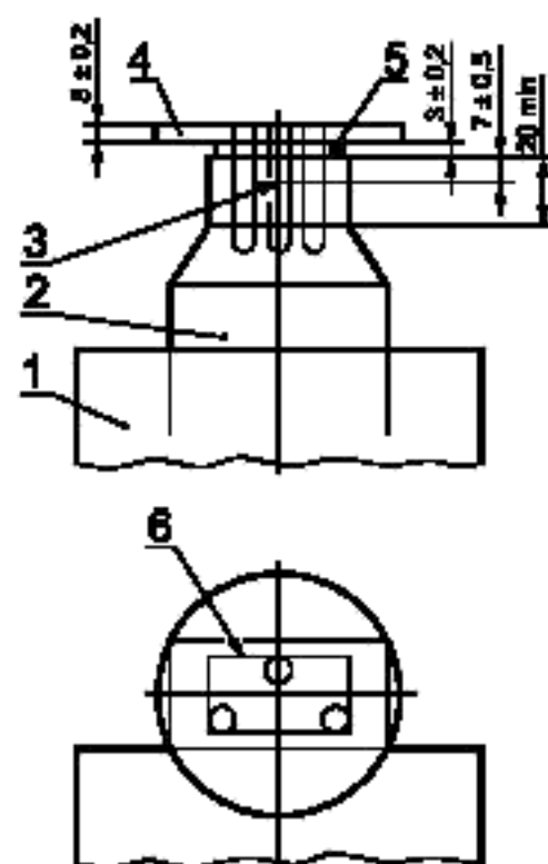
1 — нагревательный элемент; 2 — металлическая часть (деталь); 3 — термопара; 4 — изолирующая плита; 5 — прокладка; 6 — контур вилки
