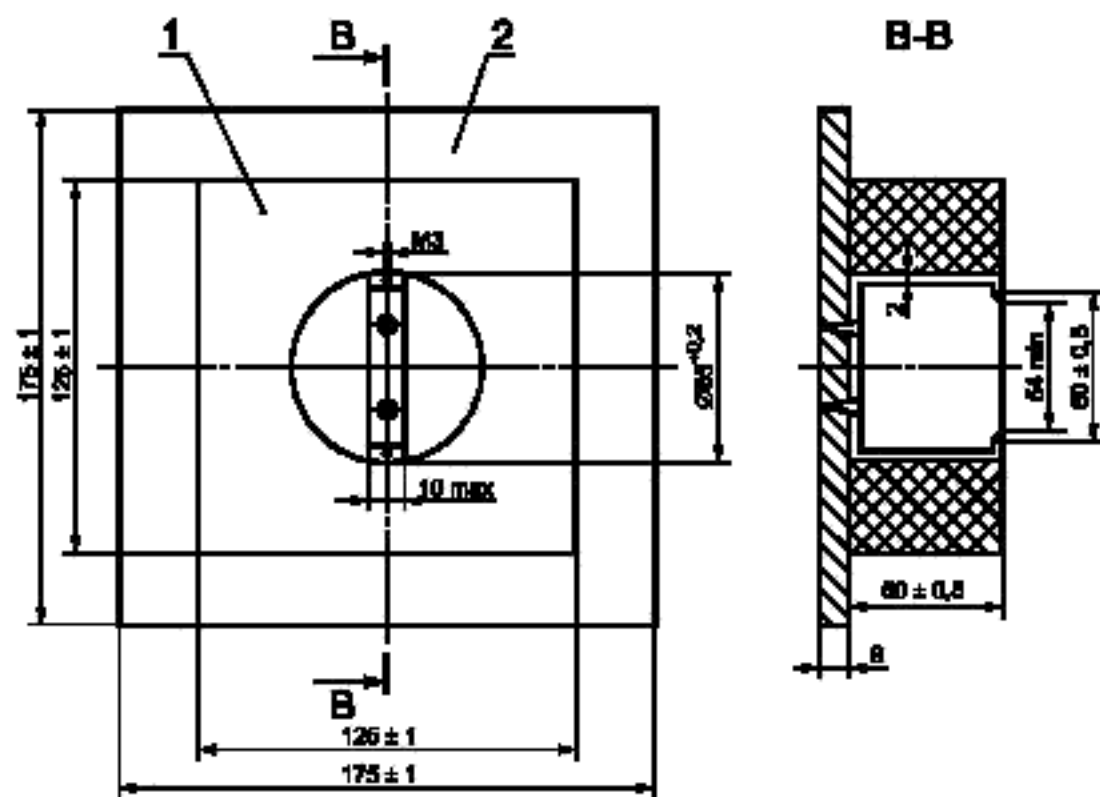
Рисунок 24 — Монтажная опора
