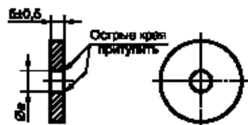
Непрямой калибр
