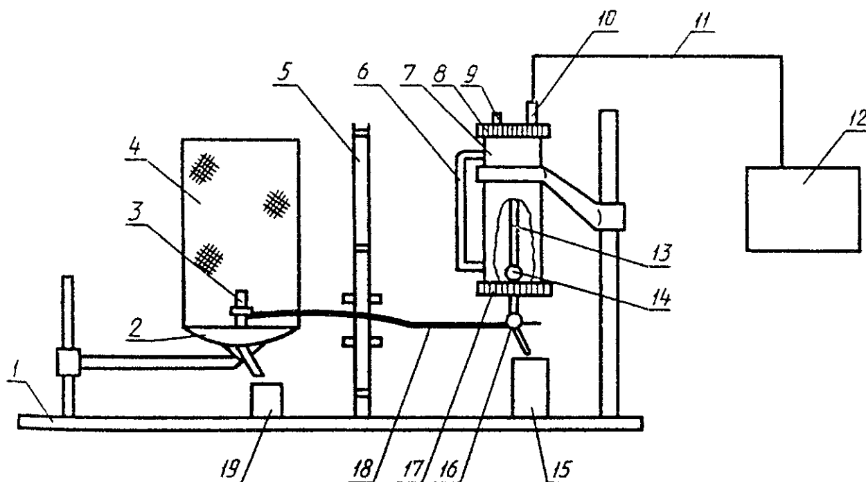
1 — основание; 2 — блок горелок; 3 — горелка; 4 — сетчатое ограждение; 5 — тепло-солирующий экран с передвижными шторками; 6 — уровнемер; 7 — заправочная емкость; 8 — верхняя крышка; 9 — винт; 10 — штуцер; 11, 18 — гибкие шланги; 11 — измерительный блок; 13 — трубка; 14 — смотровое окно; 15, 19 — стаканы; 16 — трех-ходовой кран; 17 — нижняя крышка
