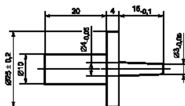
Рисунок 13 — Испытательный стержень
