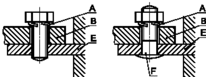
Рисунок 4 — Примеры зажимов под наконечник
