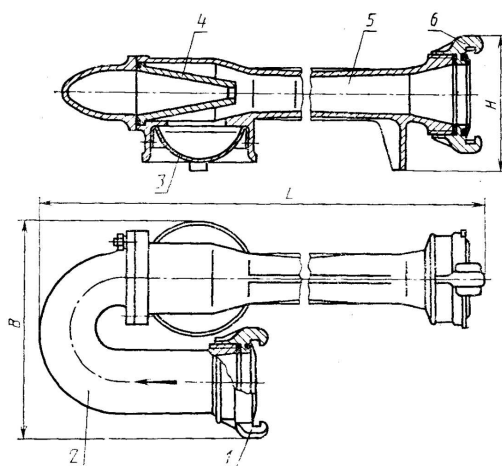
Гидроэлеватор пожарный Г-600
