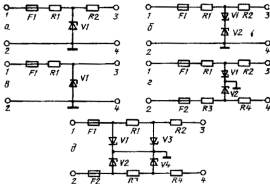
а - схема блока с балластным резистором; б - схема блока с балластным резистором для переменного тока; в - схема блока без балластного резистора; г - схема блока для переменного тока с балластными резисторами и заземленной средней точкой стабилитронов; д - схема блока для переменного тока с балластными резисторами с дублированием стабилитронов и заземленной их средней точкой; 1-2 к искроопасной цепи; 3-4 к искробезопасной цепи; V1, V2, V3, V4 - шунтирующие стабилитроны; F1, F2 - предохранители; R1, R3 - ограничительные резисторы; R2, R4 - балластные резисторы
