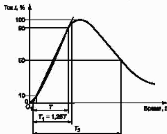
Рисунок В.6 — Волна импульсного тока 8 / 20 мкс
