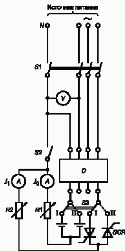
D — испытуемый АВДТ; V — вольтметр; A — амперметр (измерение действующего значения); R1 , R2 — регулируемые резисторы; S1 — многополюсный выключатель; S2 — однопольный выключатель; S3 — выключатель на два направления; SCR — тиристоры
