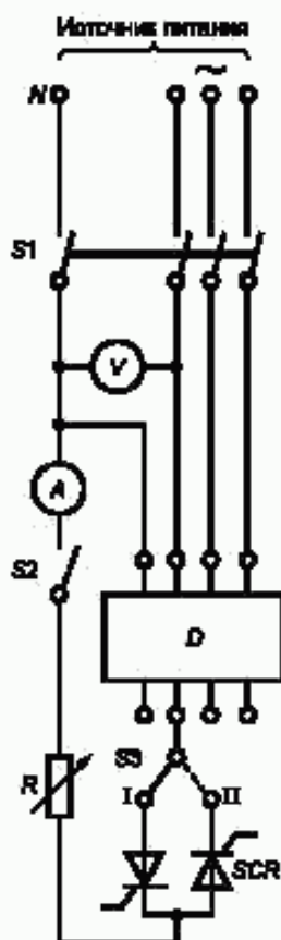
D — испытуемый АВДТ; V — вольтметр; A — амперметр (измерение действующего значения); R — регулируемый резистор; S1 — многополюсный выключатель; S2 — однопольный выключатель; S3 — выключатель на два направления; SCR — тиристоры
