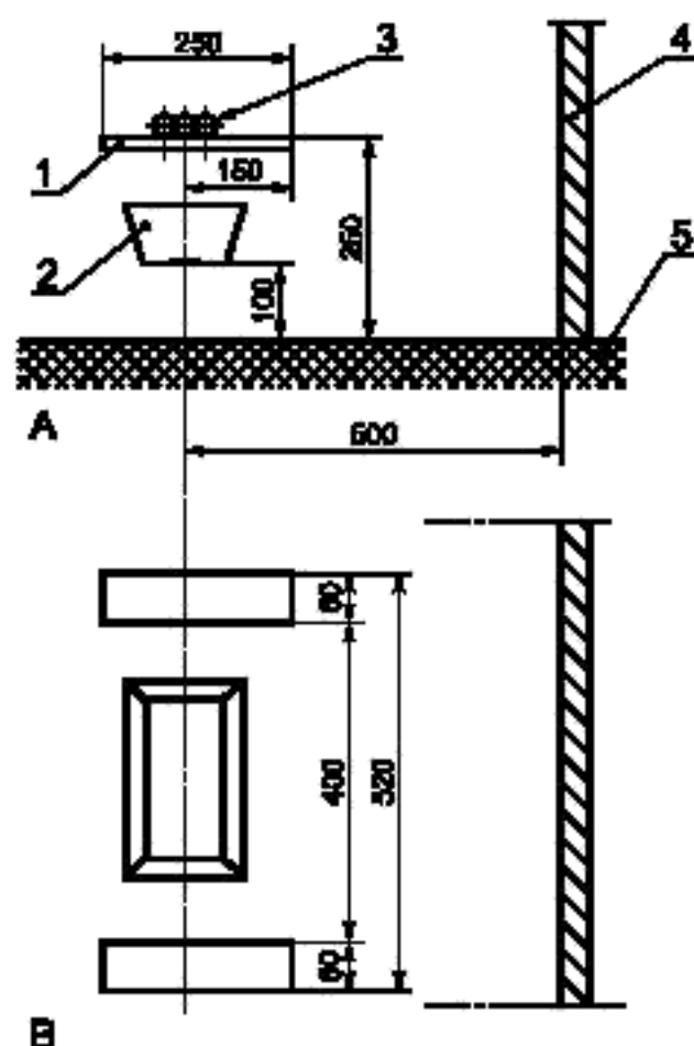
А — вид сбоку; В — вид сверху; 1 — опора; 2 — металлический поддон; 3 — испытываемый образец; 4 — задняя стенка; 5 — пол
