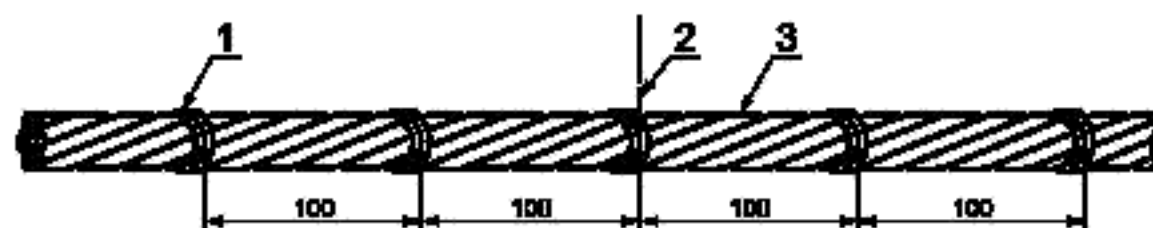
1 — проволочный бандаж; 2 — центр; 3 — число отрезков, равное семи
