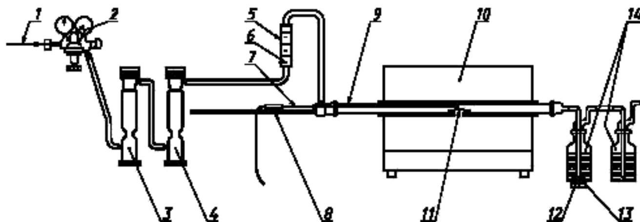
1 — сжатый воздух; 2 — редуктор; 3 — воздушный фильтр (активированный уголь); 4 — осушитель воздуха (силикагель); 5 — ротаметр; 6 — игольчатый клапан; 7 — термопара; 8 — устройство для ввода лодочки с образцом; 9 — трубка из квар- цевого стекла; 10 — печь; 11 — лодочка с образцом; 12 — магнитная мешалка; 13 — стержень магнитной мешалки; 14 — промывочные сосуды
