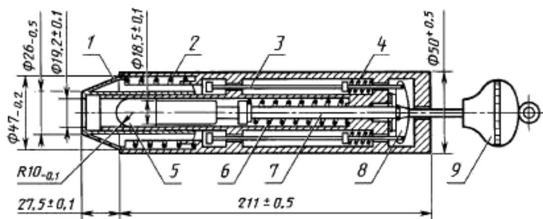
Устройство для испытания на удар
