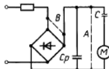
Последовательная цепь
