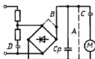
Параллельная цепь
