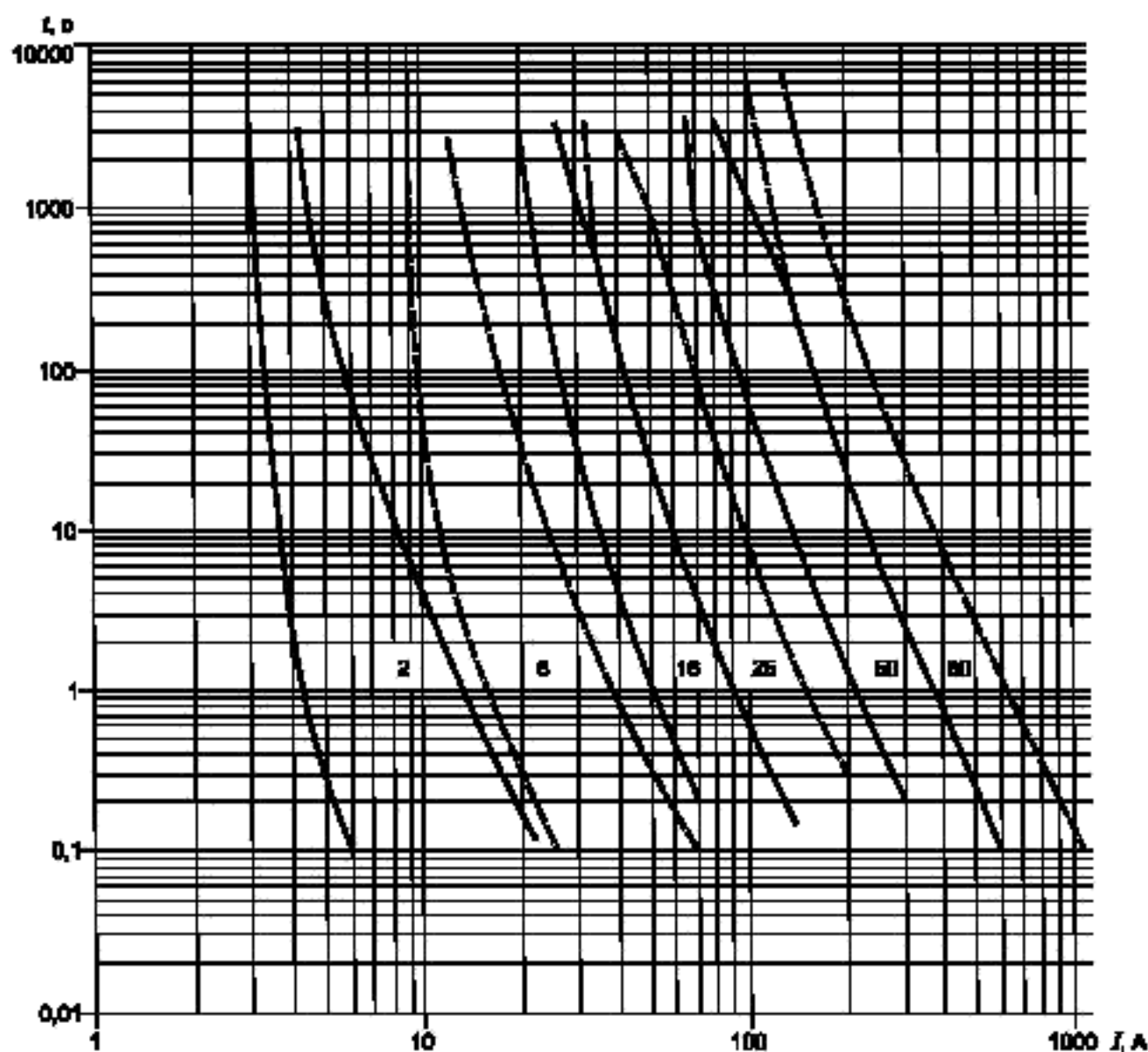
Рисунок А.1 — Время-токовые зоны для плавкого предохранителя
