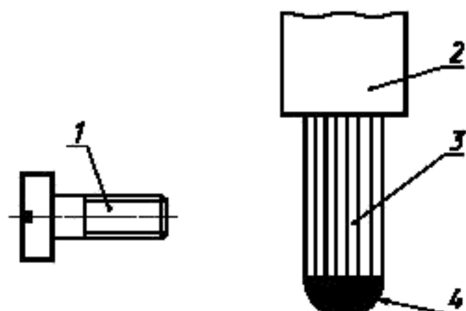
Рисунок 26 — Схема проверки безопасности зажигающего устройства
