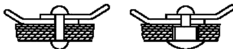
Рисунок 17 — Конструкция неразъемных соединений
