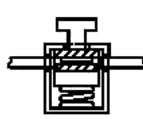
Рисунок 18 — Примеры безвинтовых контактных зажимов пружинного типа
