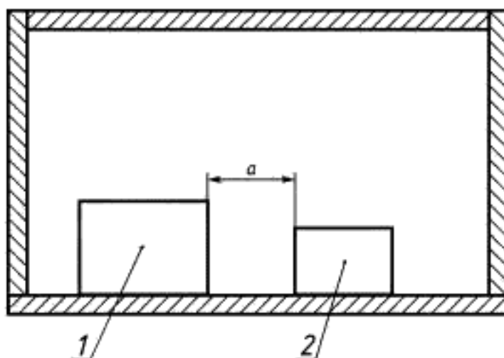
a — минимальное расстояние, указанное изготовителем; другие расстояния — в соответствии с приложением D; 1 — блок лампы; 2 — устройство управления
