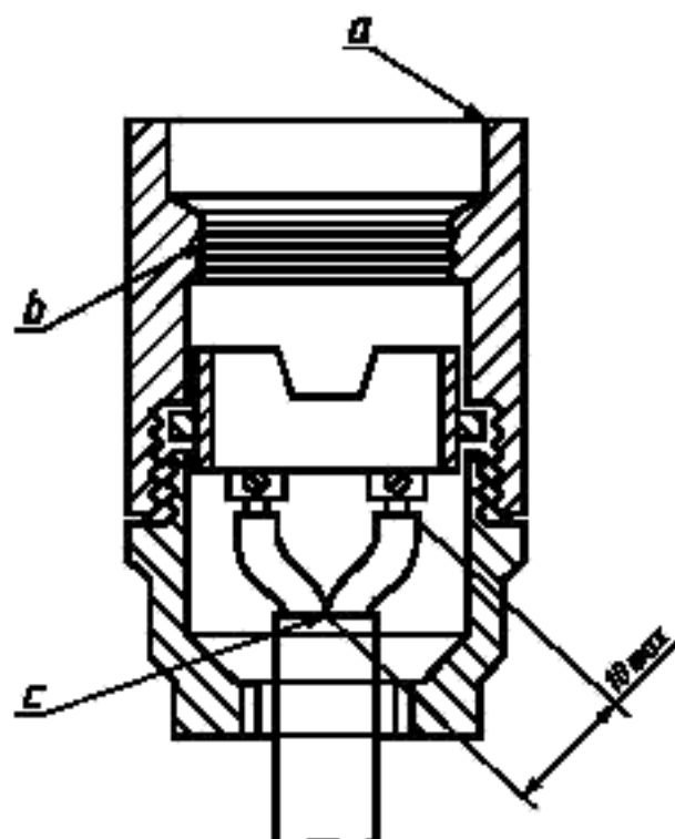
a, b, c — места расположения термопар
