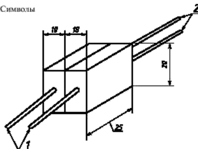
Рисунок 2 — Клемная колодка для испытания установки светильников с монтажными концами
