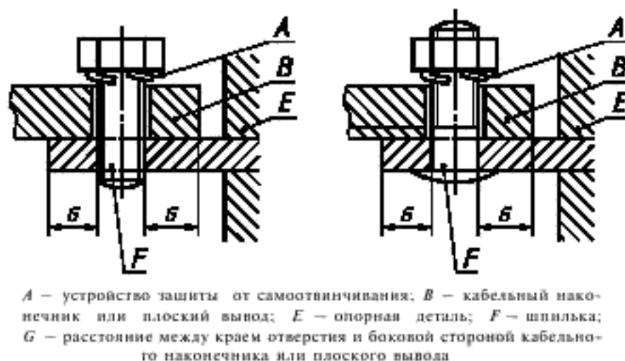
Рисунок 14 — Контактные зажимы с прижимной пластиной
