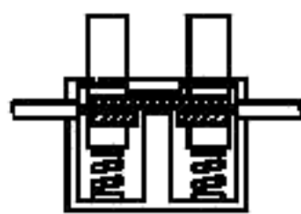
Рисунок 18 — Примеры безвинтовых контактных зажимов пружинного типа
