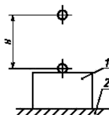
1 — образец; 2 — жесткая опорная поверхность
