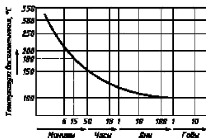
Рисунок 27 — Температура воспламенения дерева в функции времени
