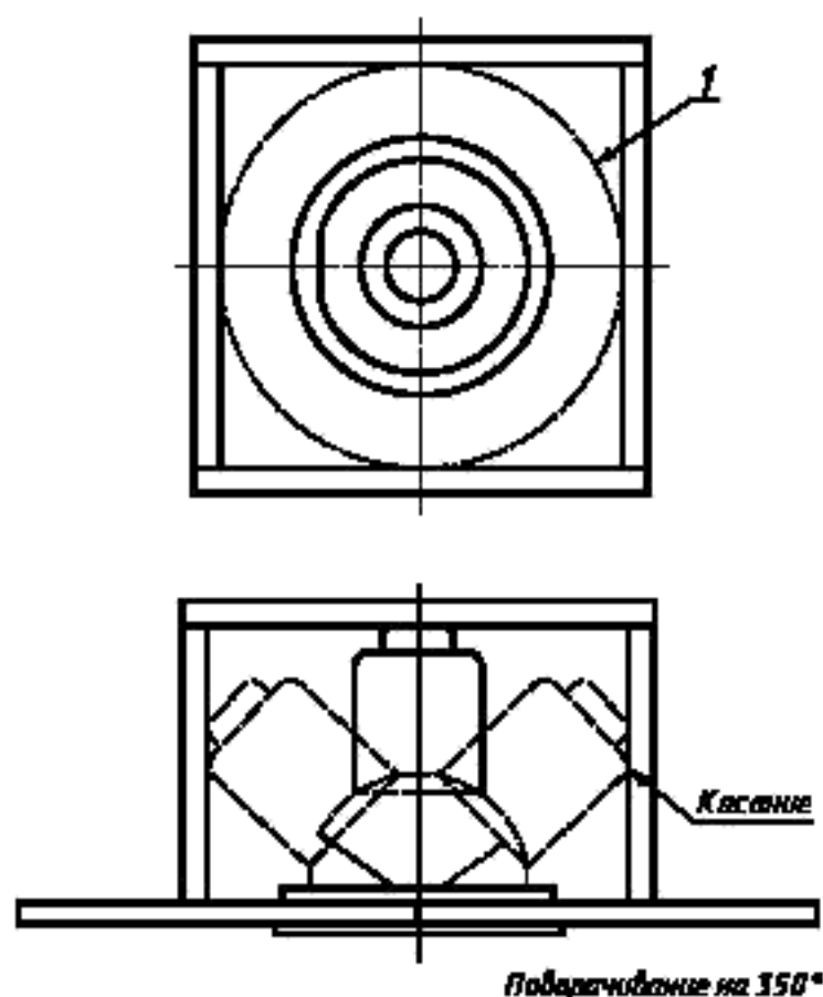
I — предельная траектория вращения поворачивающегося светильника
