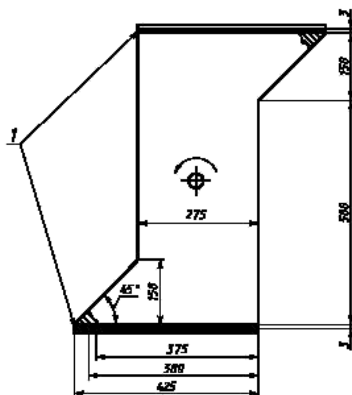
Рисунок 25 — Вращающийся барабан
