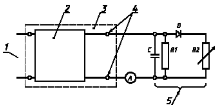
1 — сеть; 2 — ПРА, трансформатор, зажигающее устройство; 3 — светильник; 4 — место присоединения лампы; 5 — схема замещения лампы. C = 0,1 мкФ (400 В переменного тока) с пониженным затуханием; D = 100 А, обратное напряжение; R1 = 200 Ом/50 Вт; R2 = 0-100 или 0-1, 1-10, 10-50, 50-100 Ом, регулируемое
