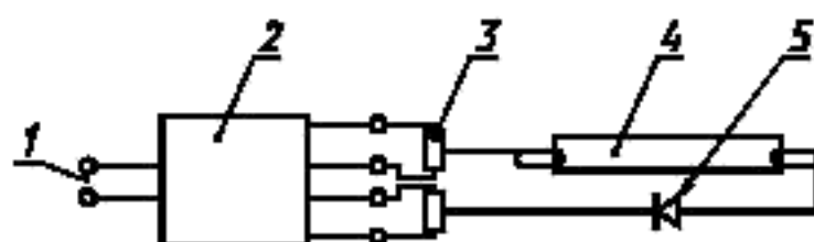
1 — сеть; 2 — испытуемый ПРА; 3 — резистор; 4 — лампа; 5 — выпрямитель
