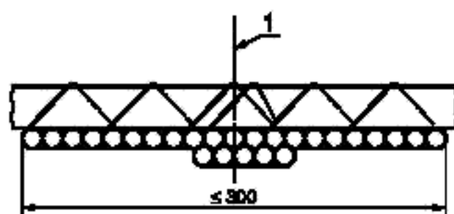
Рисунок 1 — Кабели, закрепленные на передней стороне стандартной лестницы без зазора (комплекты отрезков кабелей находятся в контакте)
