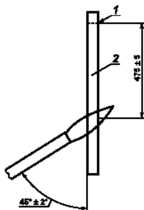
1 — нижний край верхней опоры; 2 — образец
