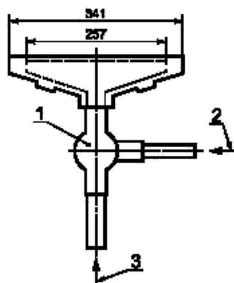
a — одиночная горелка, используемая при стандартной лестнице
