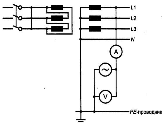
Рисунок D.2. Схема измерения (метод 2)
