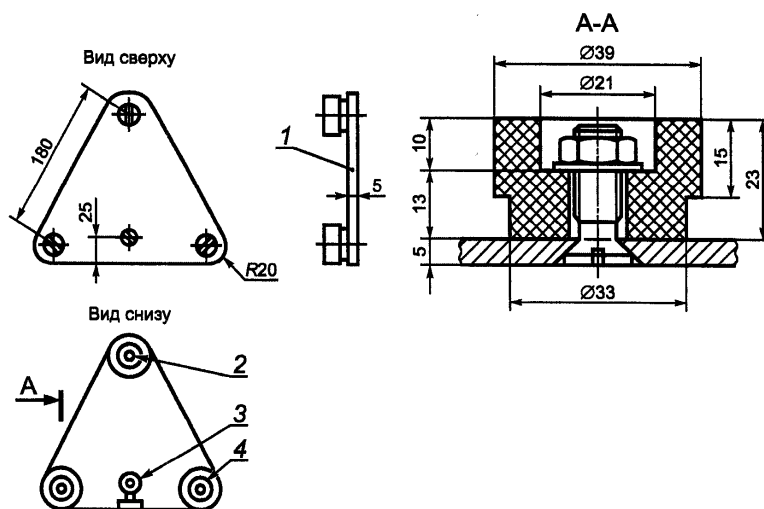
1 - алюминиевая пластина; 2 - винт с шайбой и гайкой; 3 - клемма; 4 - контактная ножка из проводящей резины Рисунок А.1. Измерительный электрод 1
