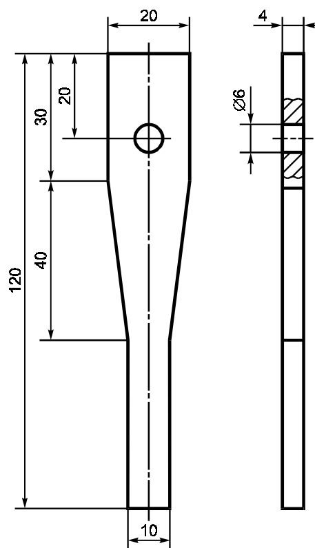
Рисунок 1.3 — Стальная пружина
