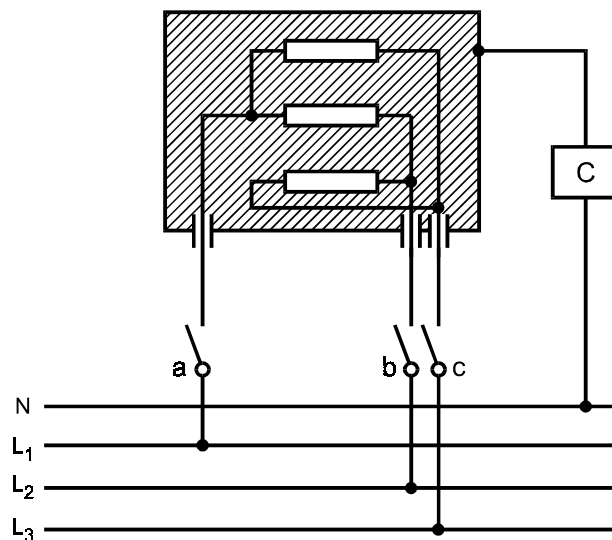
Рисунок 4 — Схема измерения тока утечки при рабочей температуре для трехфазных приборов, кроме приборов класса II
